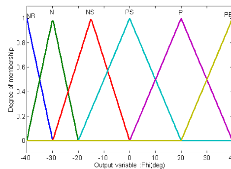
Fig. 12. MF( \phi )
